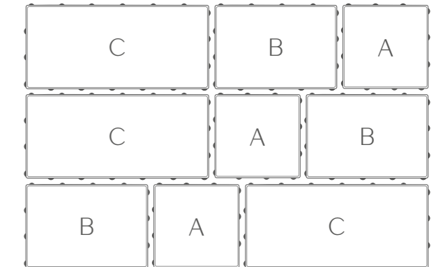
Układ kostek w warstwie
