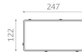
Wymiary kostki brukowej DREWBET® HOLLAND BIG MF 60
