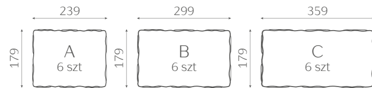
Wymiary kostki brukowej DREWBET® TROTUAR MF 60
